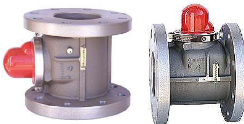
شکل ۲۱-۷-۵- شیر خودکار قطع جریان گاز حساس در مقابل زلزله قائم و افقی فلنجی
